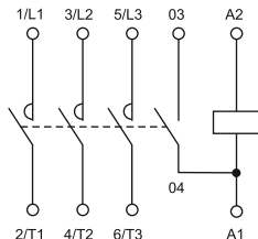
Рисунок 1 – Схема электрическая контакторов
