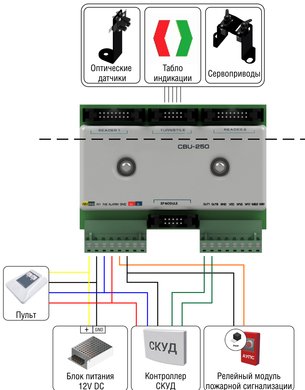
Рисунок 17 – Схема подключений ЦБУ турникета
