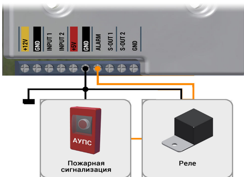
Рисунок 20 - Подключение АУПС к турникету
