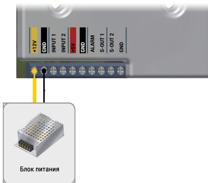
Рисунок 18 - Подключение питания к турникету
