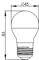
Рисунок 13 – Лампа LED-G45, 9 Вт, цоколь E27
