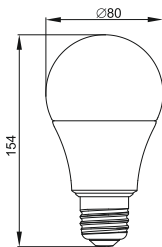
Рисунок 33 – Лампа LED-A80, 25 Вт цоколь E27
