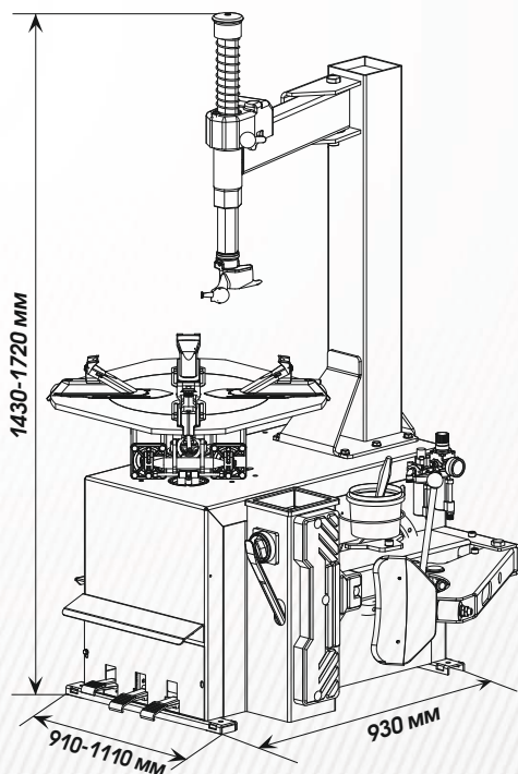
Рисунок 4 Установка стэнда
