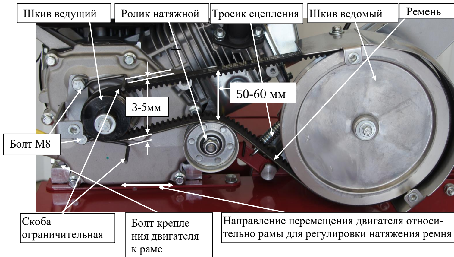
Рис.6 Схема натяжения ремня.
