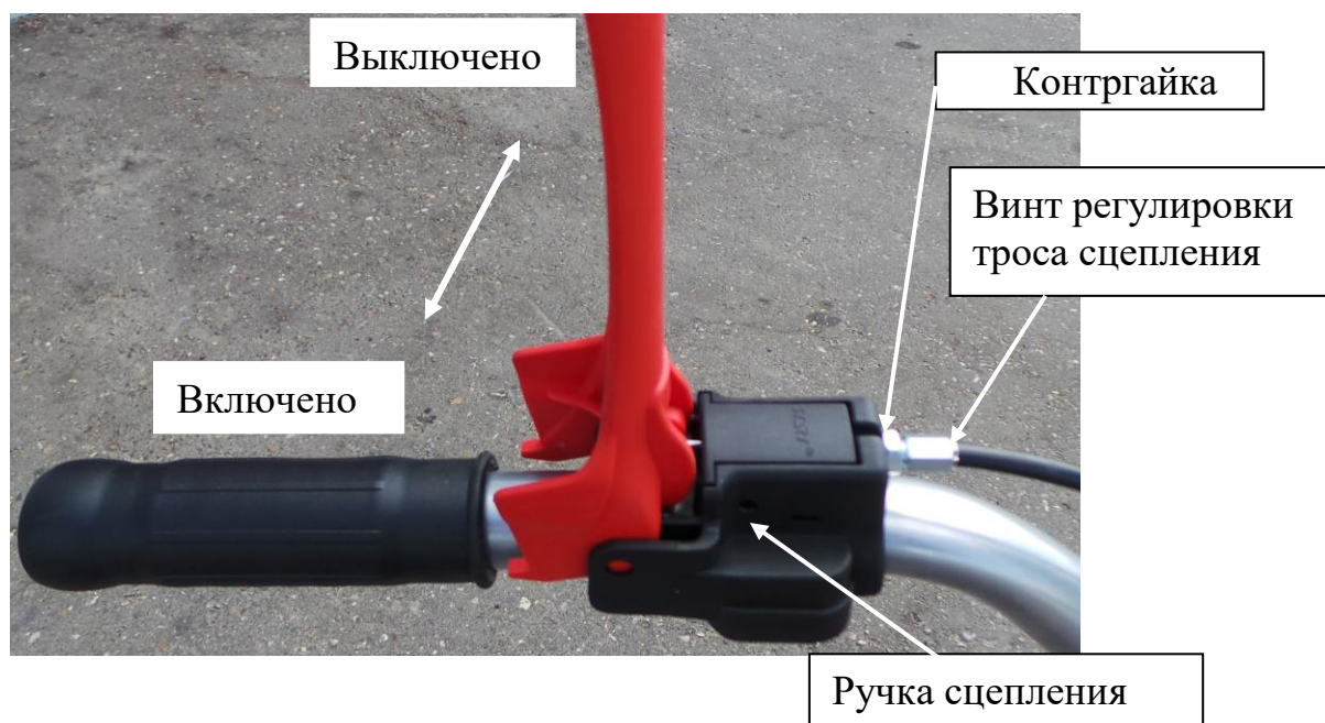
Рис.8 Ручка сцепления в комплекте с тросом.
