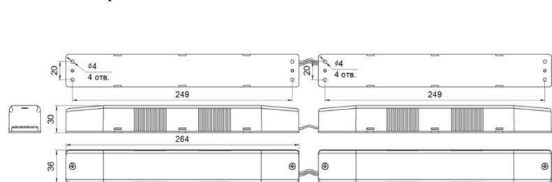
Рис. 9 Блок аварийного питания BS-STABILAR2-81-B2-LED BOX IP30
