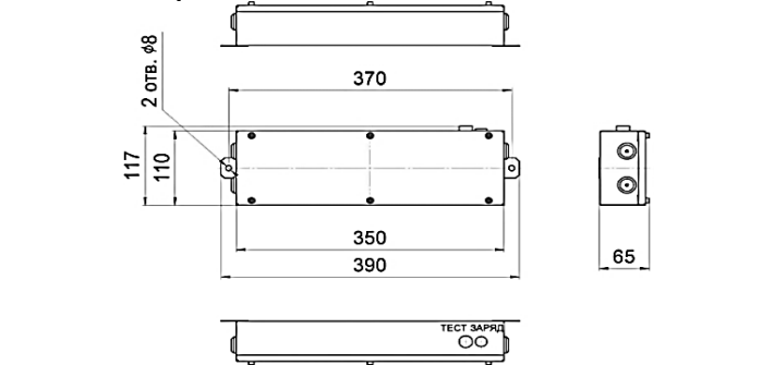
Рис. 10 Блок аварийного питания BS-STABILAR2-81-B2-LED BOX IP65
