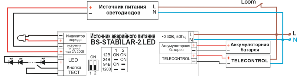
Рис. 1 Схема подключения BS-STABILAR2-81-B2-LED для аварийного светового прибора в универсальном режиме:
