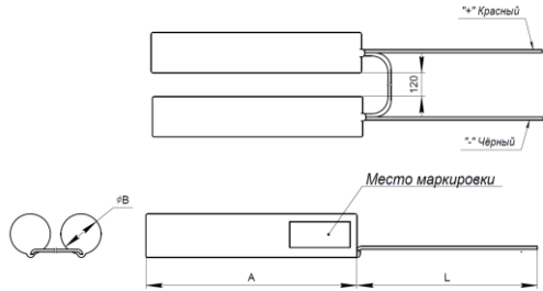
Батарея BS-3+3HRHT14/50-1,6/A-HB500-0-1 а18279
