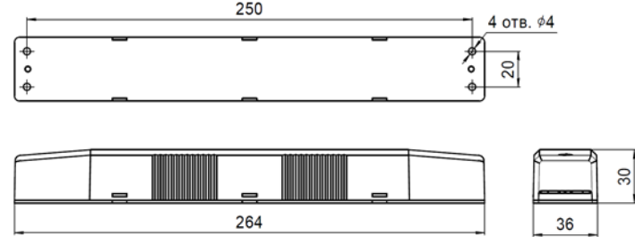
Рис. 7 Блок аварийного питания BS-STABILAR2-81-B2-LED
