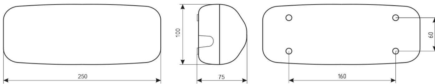
Рис. №3 Габаритный чертёж.
