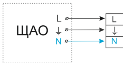
Рис. №2 Схема подключения к групповой цепи управления.
