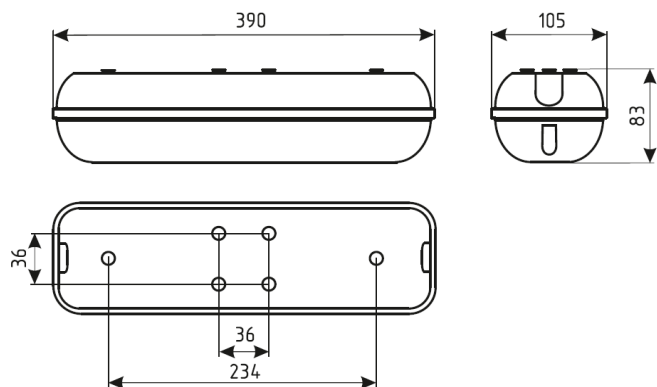
Рис. №2 Габаритный чертёж.
