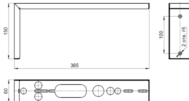
Рис. №3 Кронштейн BS-K-3
