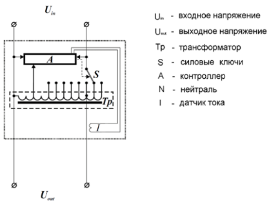
Рисунок 3. Функциональная схема стабилизатора
