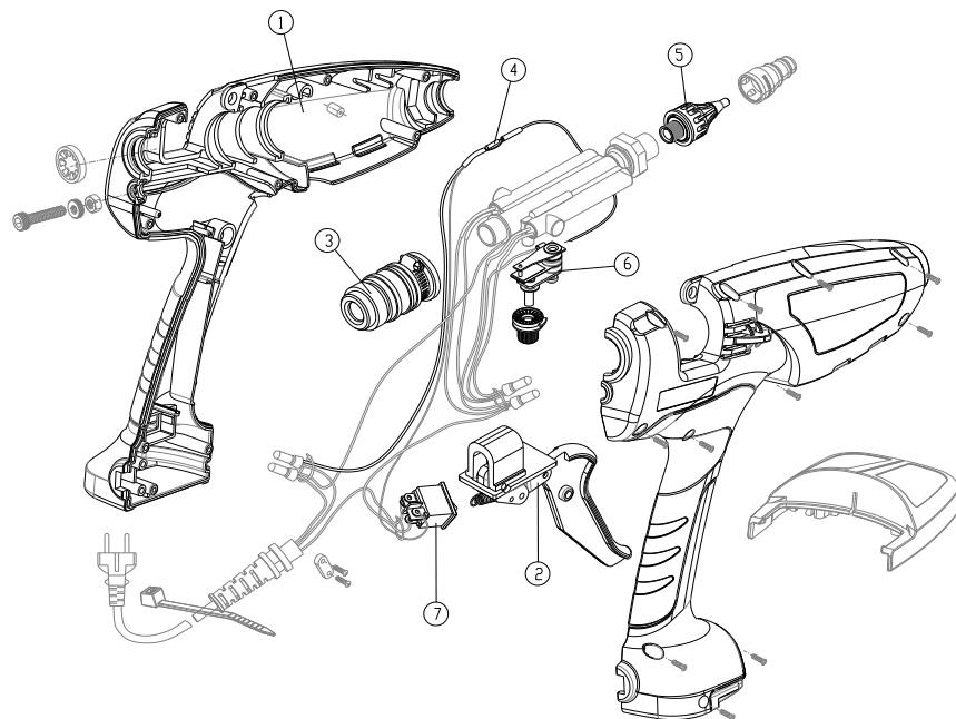
СХЕМА ТЕРМОКЛЕЕВОГО ПИСТОЛЕТА
