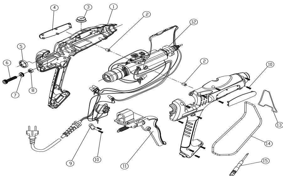
СХЕМА ТЕРМОКЛЕЕВОГО ПИСТОЛЕТА
