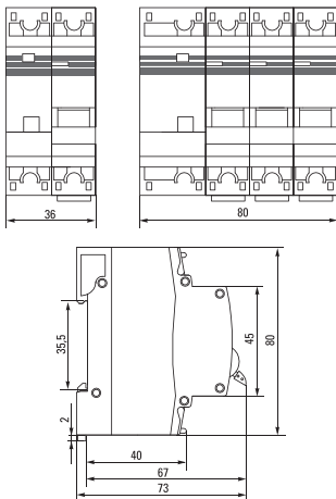
Рисунок 2. Габаритные и установочные размеры АД-32S (селективный) – двухполюсный и четырехполюсный.
