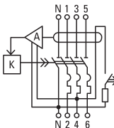
Рисунок 1. Принципиальные схемы подключения АД-32S (селективный).
