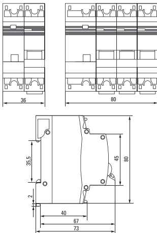
Рисунок 5. Габаритные и установочные размеры АД-32 (тип А) – двухполюсный и четырехполюсный
