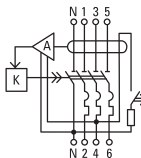
Рисунок 1. Принципиальные схемы подключения АД-32 (тип А)
