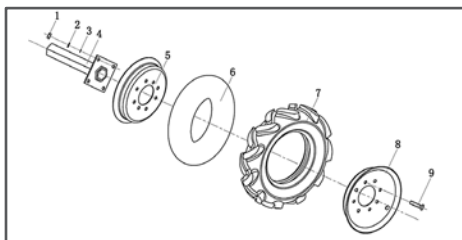
Рис. 3 Установка колеса на Мотокультиватор 1.Гайка
