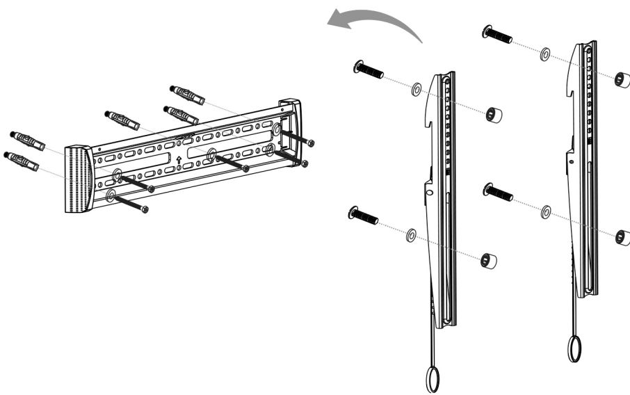
Assembly scheme Сборочный чертёж
