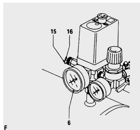
Внешний вид и составные части компрессора (Рис А)
