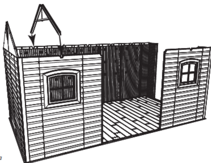
Capriata lato esterno / Grindă laterală externă / Внешняя боковая ферма
