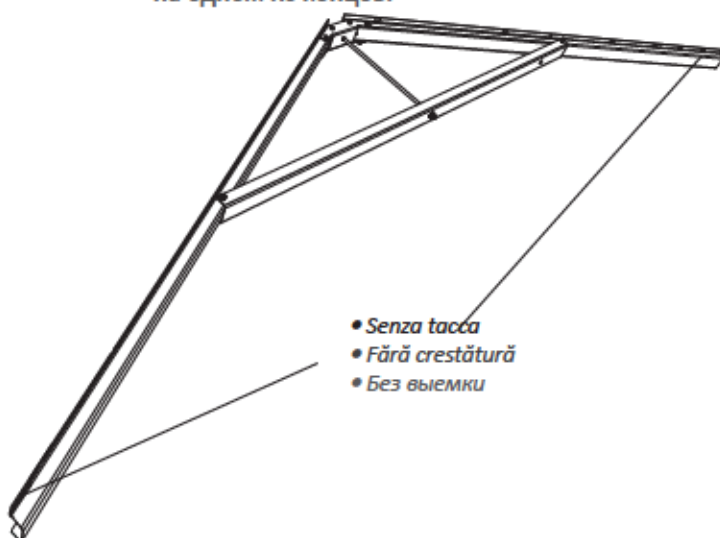
Capriata lato esterno / Grindă laterală externă / Внешняя боковая ферма
