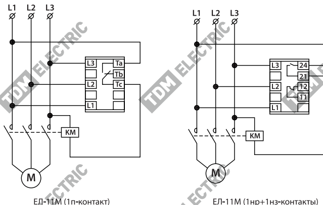
Рисунок 3. Схема подключения реле ЕЛ-11М к электрической сети
