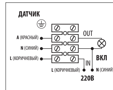
Рис 1. Схема подключения датчика
