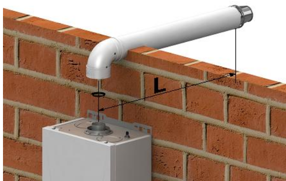
Рис. 3 Схема присоединения коаксиального дымохода \varnothing 100 / \varnothing 60 (мм) к котлу и установка диафрагмы
