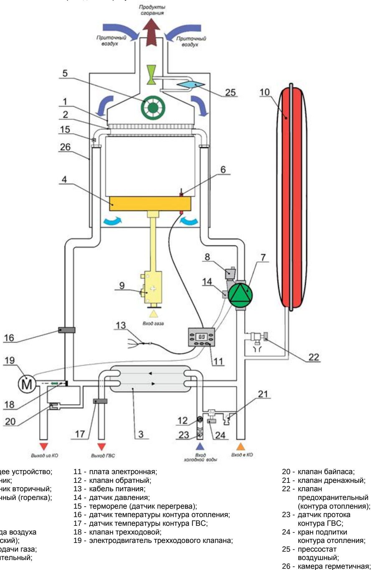
Рис. 7 Функциональная схема котла
