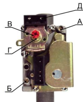
Рис. 6 Регулятор подачи газа
