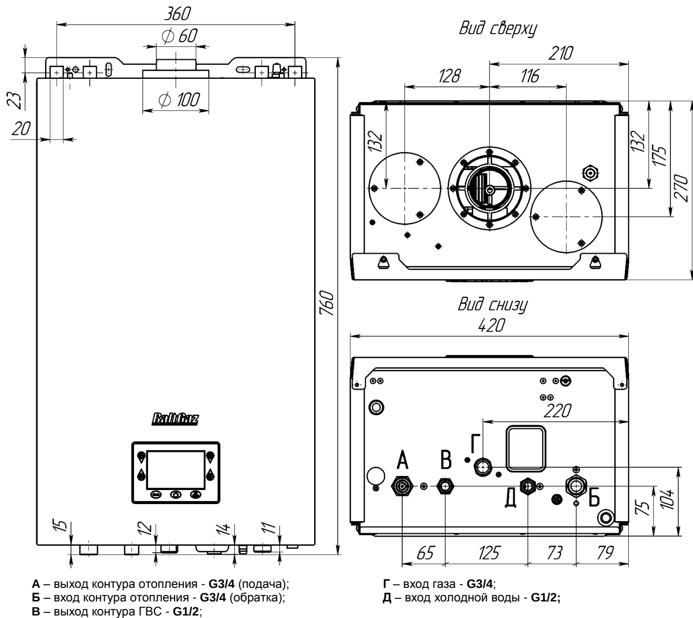
Рис. 1 Габаритные и присоединительные размеры котлов
