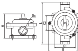
Рис. 5 Пакетные выключатели серии ПВ – Исполнение в силуминовом корпусе
