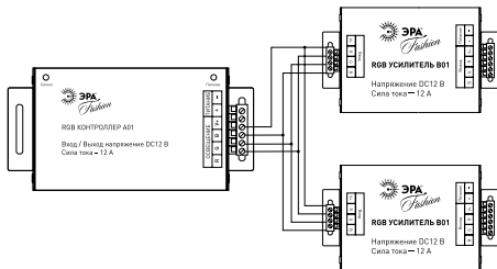
Рис.4. Параллельная схема включения.
