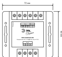
Рис. 2. Габаритные размеры усилителя RGBpower-12-B02 .
