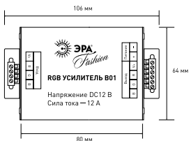
Рис. 1. Габаритные размеры усилителя RGBpower-12-B01 .
