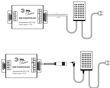
Рис.6. Варианты подключения источника питания к усилителю RGB сигнала
