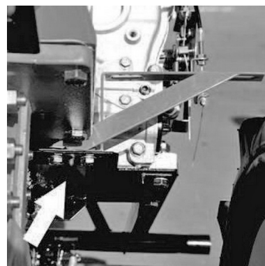
Шаг 12. Прикрепить кронштейны крепления защитных кожухов к раме двигателя
