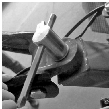
Шаг 5. Установите руль, для чего совместите зубья его половины зубчатого седла с зубьями соот- ветствующей половины зубча- того седла на рулевой колонке. Зафиксируйте требуемое поло- жение руля, зажимая зубчатое седло руля зажимной головкой.
