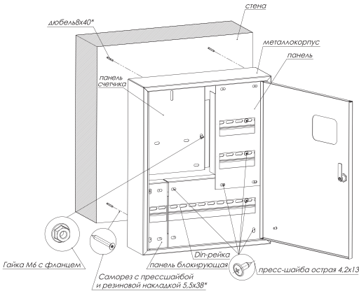
Рис.1. Схема монтажа
