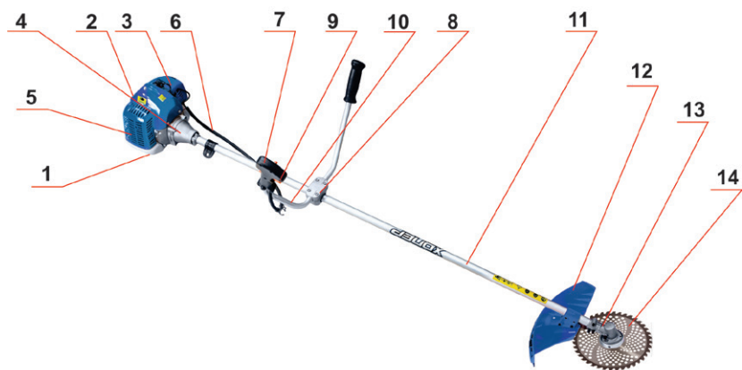
Рис. 2. Расположение основных элементов бензотриммера:
