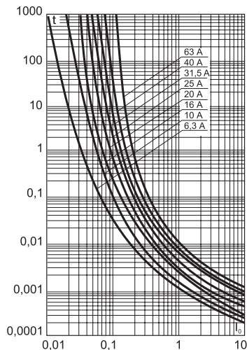
Рисунок В.2 – Преддуговые время-токовые характеристики при напряжениях 380 и 500 В переменного тока
