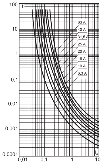
Рисунок В.5 – Преддуговые время-токовые характеристики при напряжении 220 В постоянного тока
