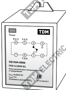
Рисунок 1. Реле контроля фаз РКФ-3х380В-8Ц
