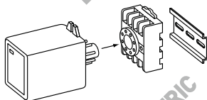
Схема установки реле ПКФ на DIN-рейку
