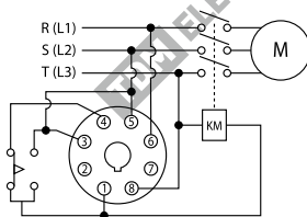
Рисунок 4. Схема подключения реле ПКФ к электрической сети
