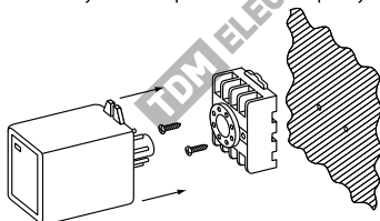
Схема установки реле ПКФ на монтажную плоскость
