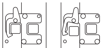
Рис. 3. Положения защелки
