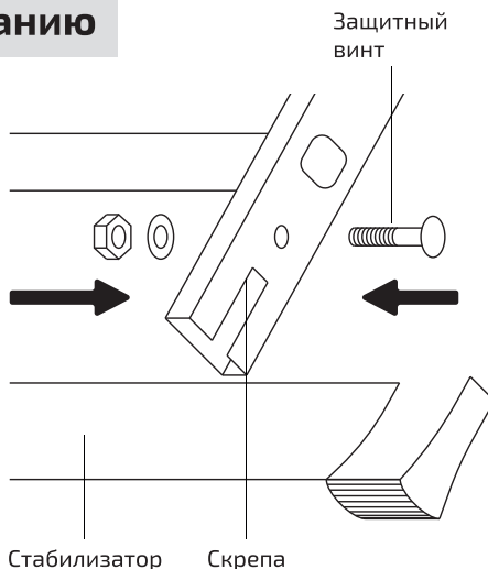
Рис. 2. Закрепление траверсы устойчивости
