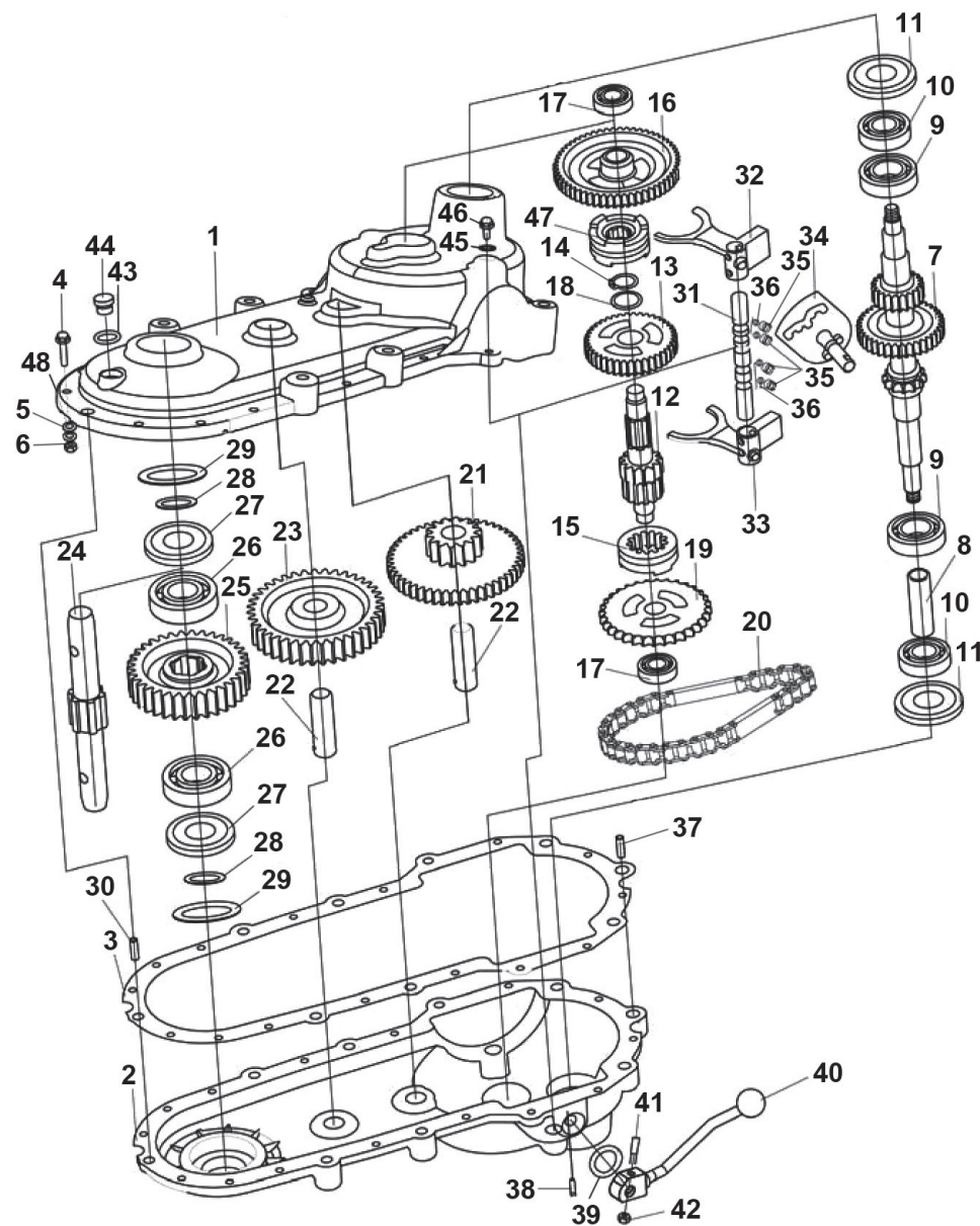
Схема сборки № 2
