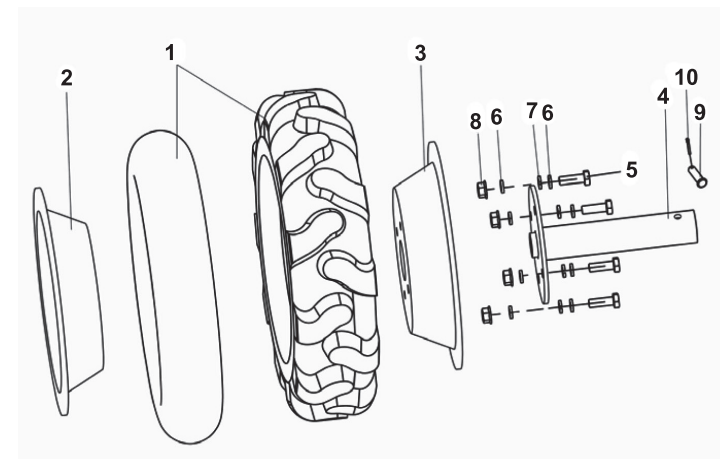
Схема сборки № 6
