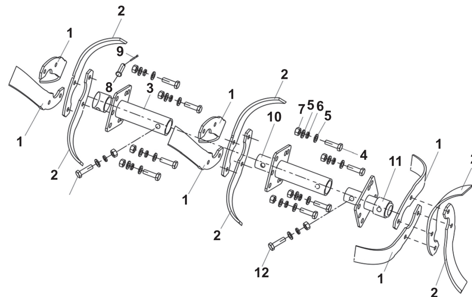
Схема сборки № 6
