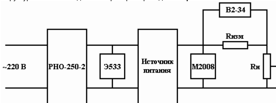
Рисунок 2. Структурная схема измерения нестабильности выходного тока при изменении напряжения питающей сети в режиме стабилизации тока
