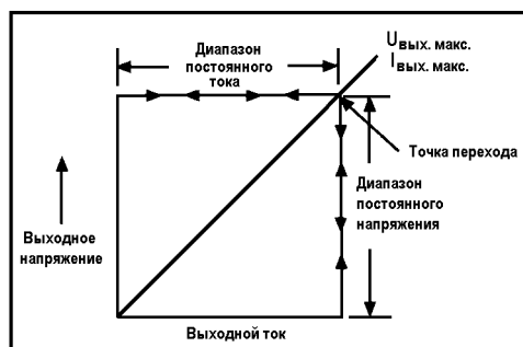
Рисунок 6.1. Вольтамперная характеристика источника
