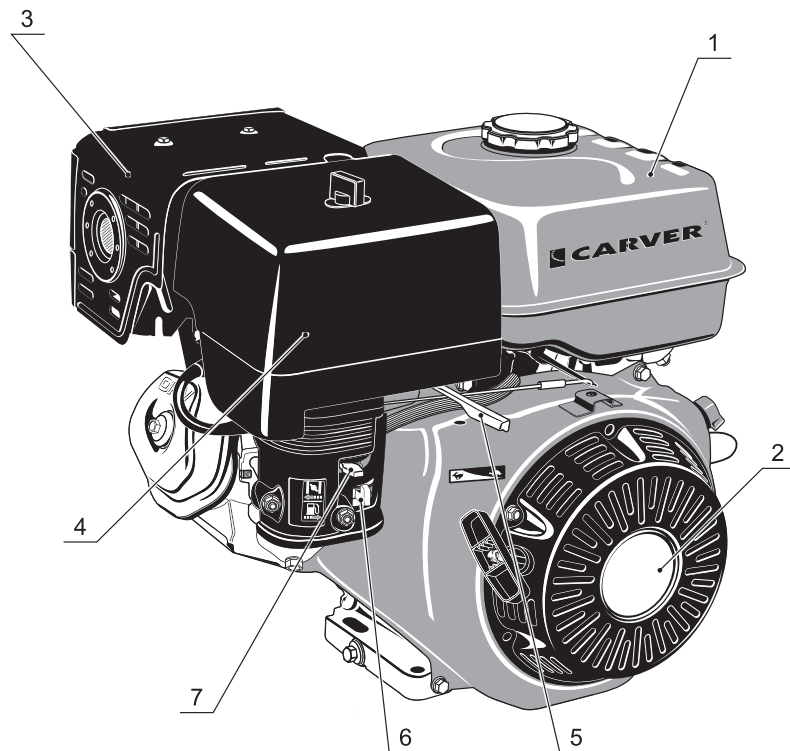
Рис. 1. Двигатель в сборе
