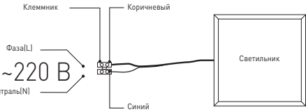
Рис.1. Схема подключения светильника к сети 220В.
