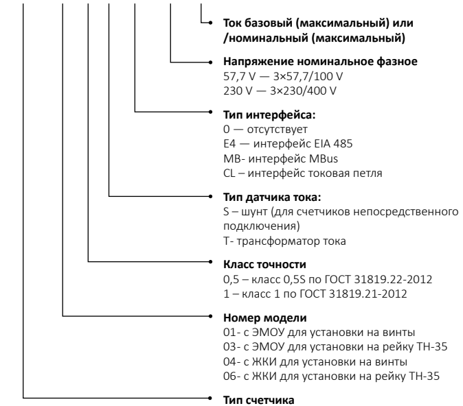
Рисунок 1 — Структура условного обозначения счетчиков НЕВА 3
