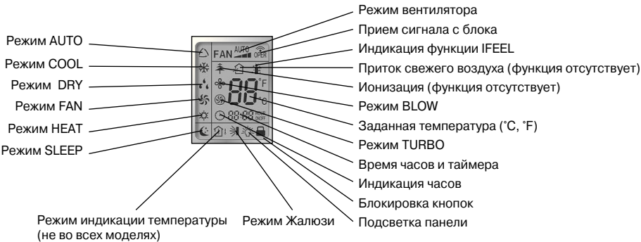
Рис. 5.1.1 Индикация пульта
