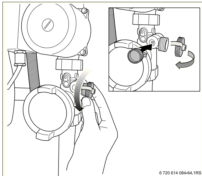
Рис 32 Крышка крана заполнения и слива
