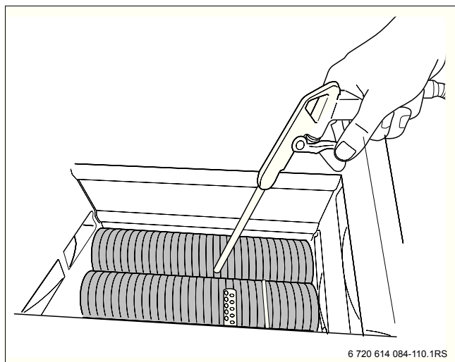
Рис 73 Чистка теплообменника
