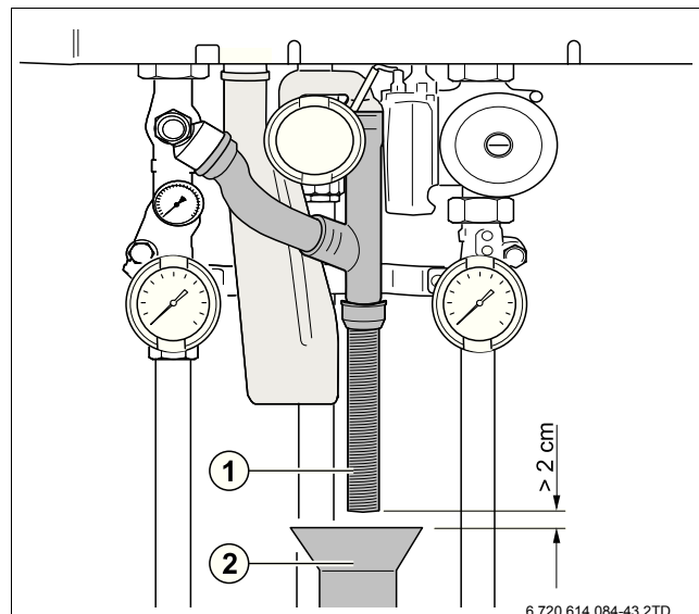
Рис 16 Минимальное расстояние до гофрированного шланга
