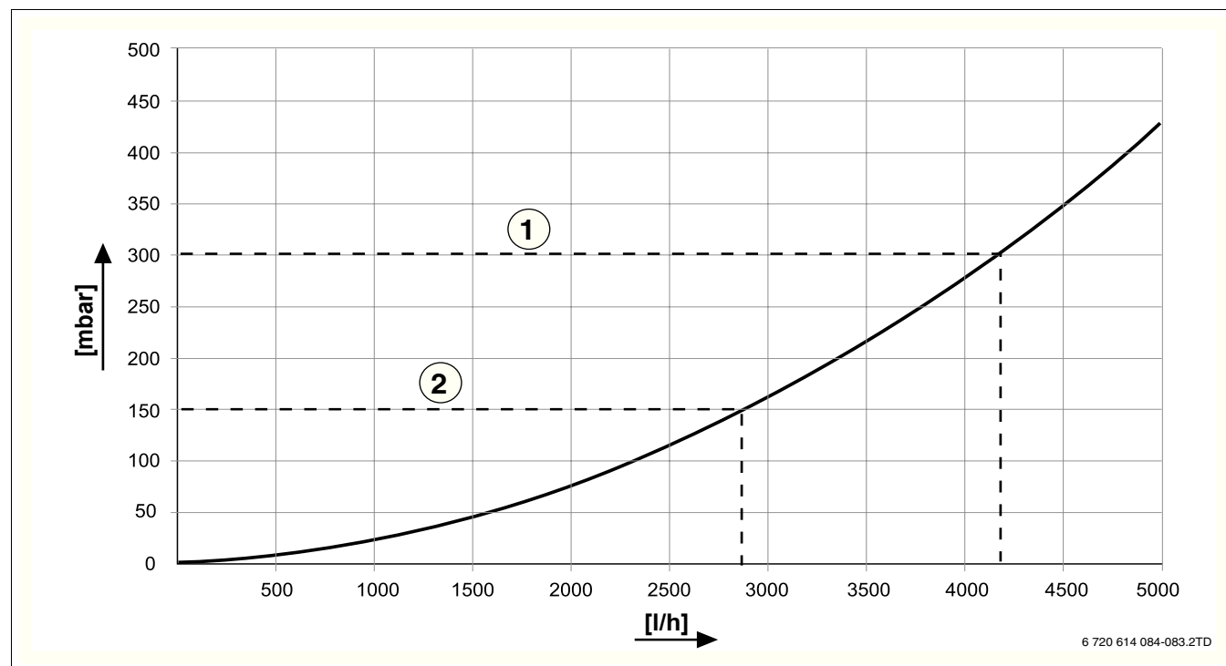
Рис 84 Характеристика сопротивления
