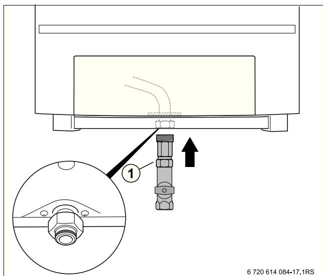
Рис 12 Подключение газа
