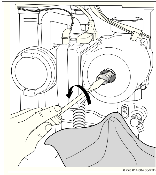
Рис 37 Удаление воздуха из насоса
