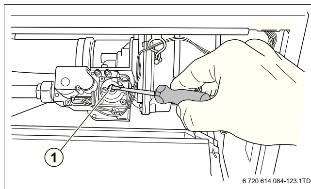
Рис 45 ZBR 65-2: регулировочный винт регулировки соотношения газ/воздух
