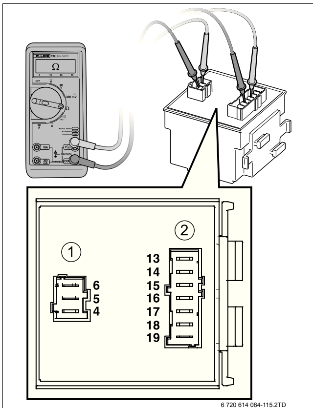
Рис 82 Проверка трансформатора
