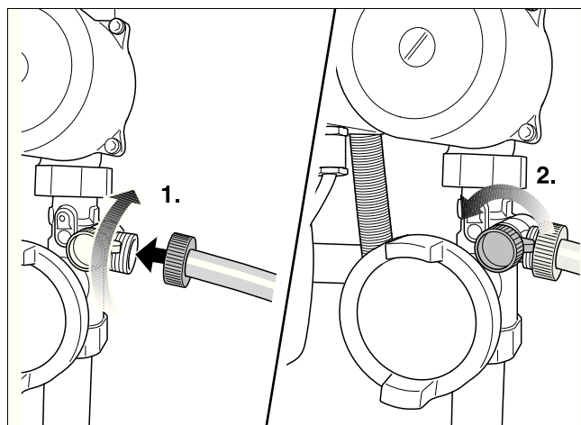
Рис 33 Подсоединение шланга
