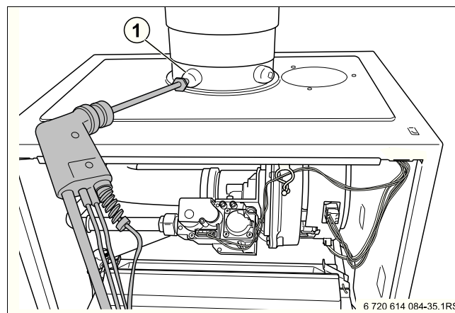
Рис 46 Точка замера дымовых газов
