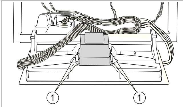
Рис 81 Демонтаж трансформатора
