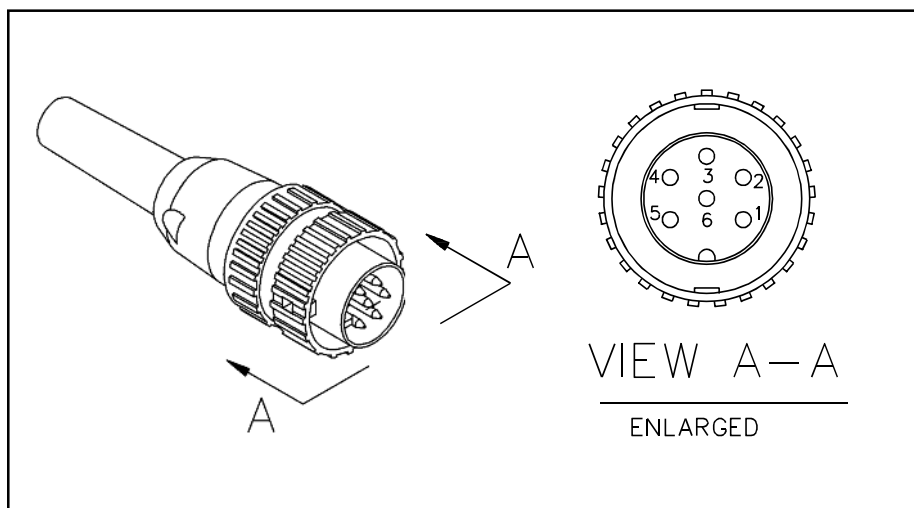
Распиновка разъема
