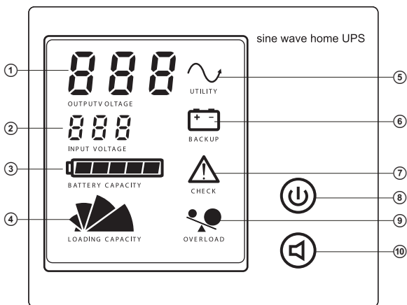
Fig. 1. UPS display
