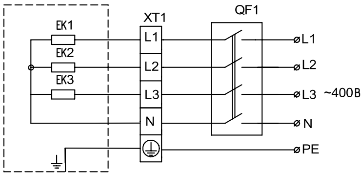
Схема электрическая принципиальная инфракрасных обогревателей ВІН-АР4-3.0 при подключении к электрической сети через автоматический выключатель.
