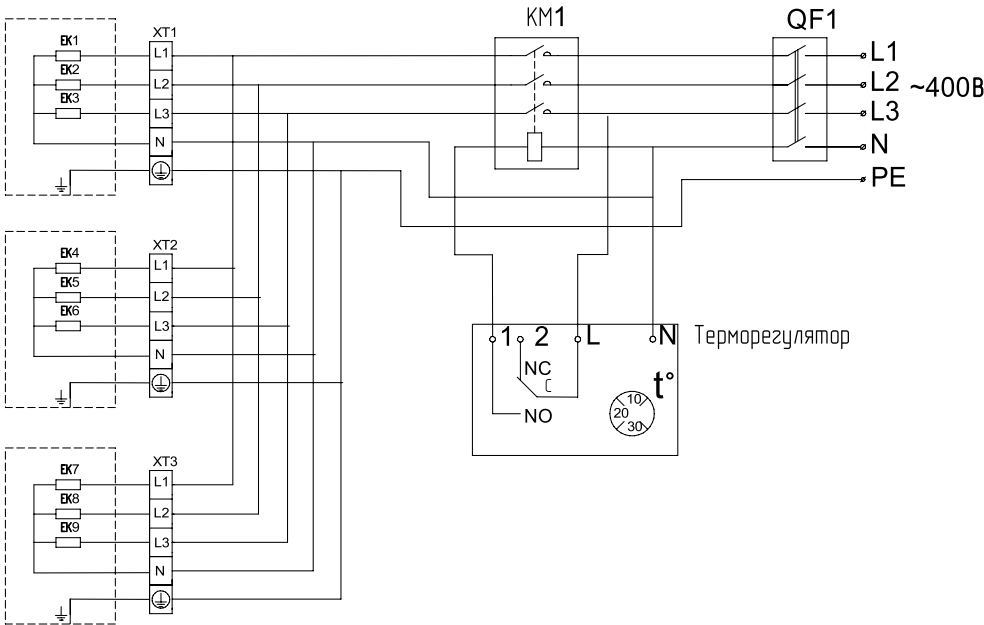
Схема электрическая принципиальная инфракрасных обогревателей ВІН-АР4-3.0 при групповом подключении к электрической сети.
