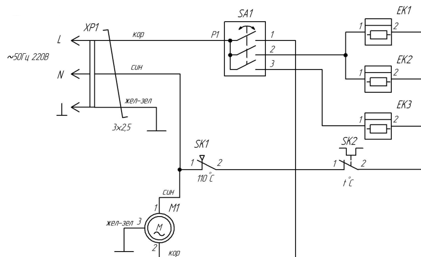
Схема коммутации переключателя SA1
