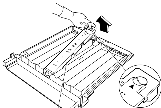
Устройство разряда стримера
