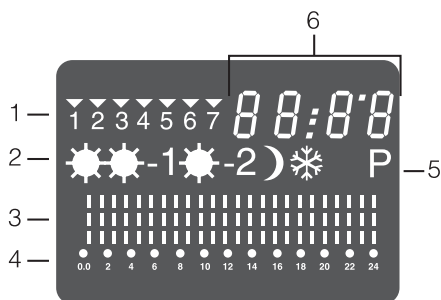
Рис. 5. Дисплей
