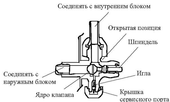
Схема четырех-ходового клапана
