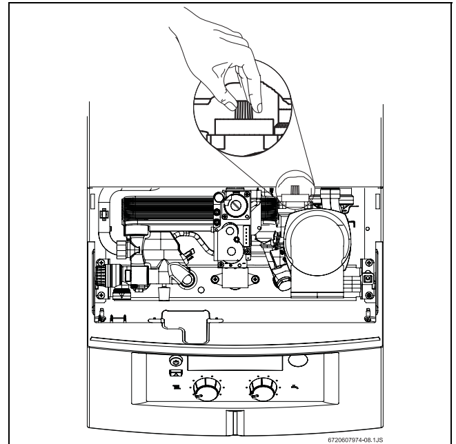
Рис 17 Воздухоотводчик
