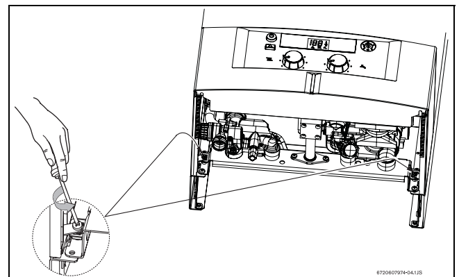
Рис 8 Расположение винтов
