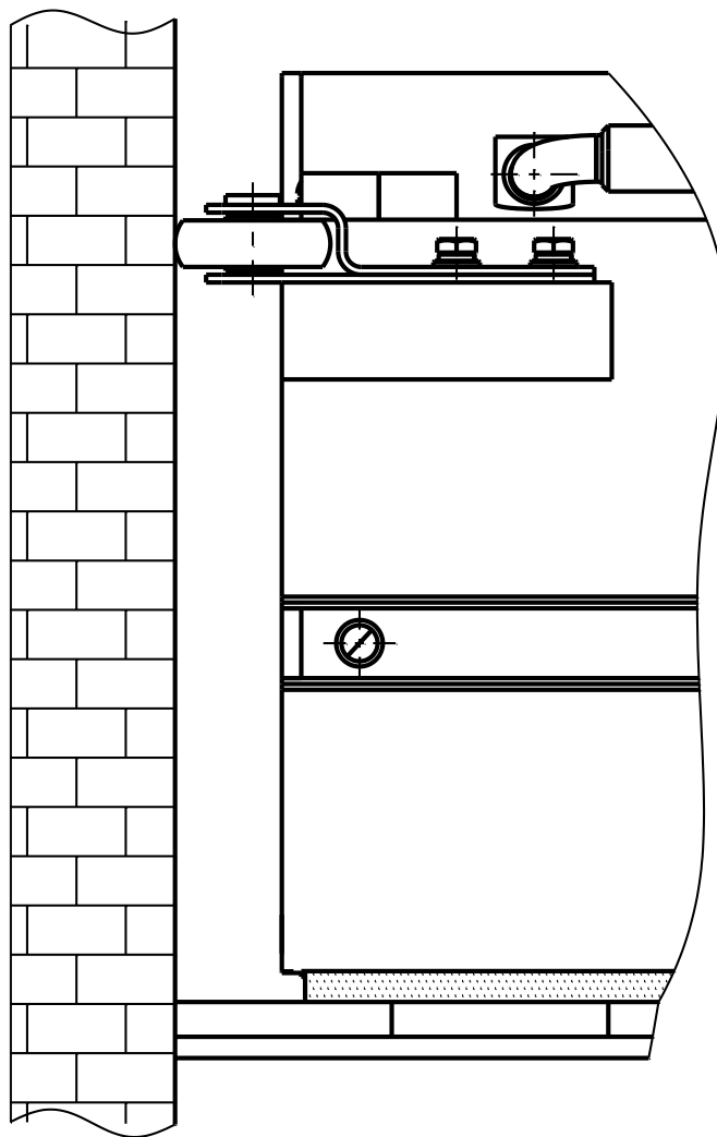
Рисунок 5 – Схема установки упора
