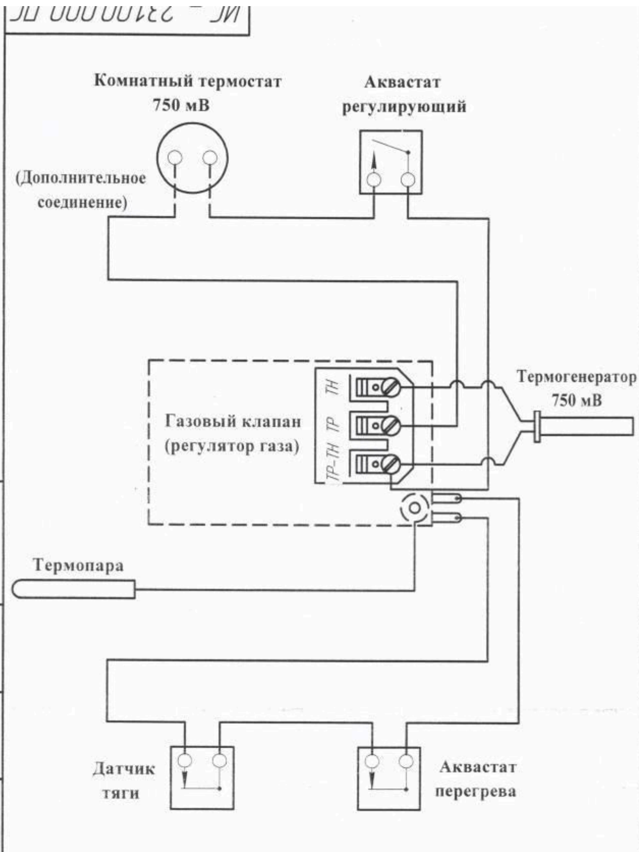
Рис. 3 Схема Электрических соединений.
