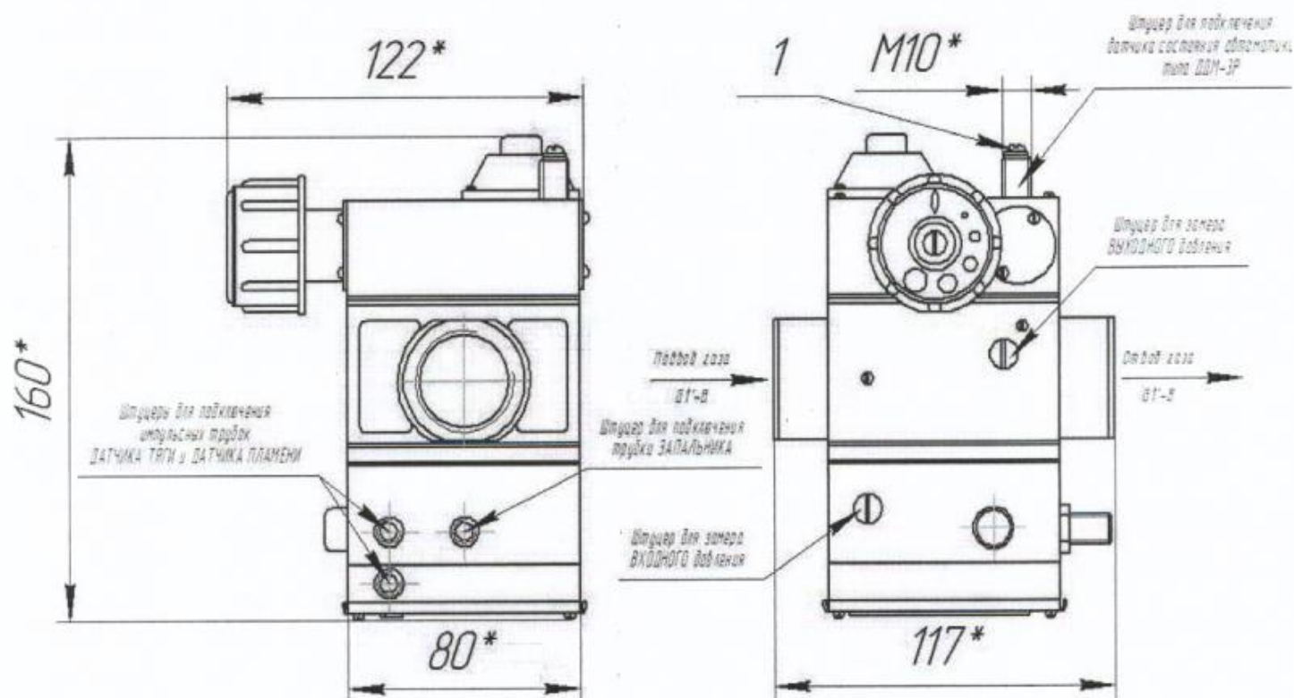
Рис. 2Б. Схема расположения точек подключения блока автоматики.
