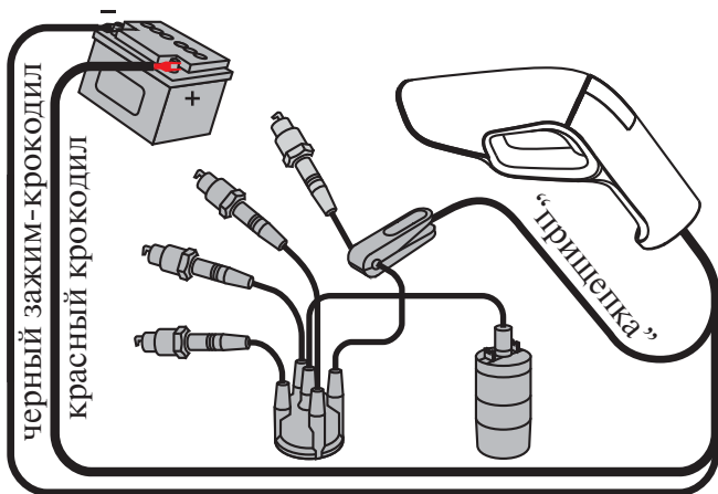
Рис. 1 - Схема подключения
