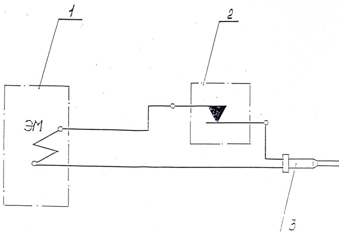
Рис. 3 Схема электрическая
