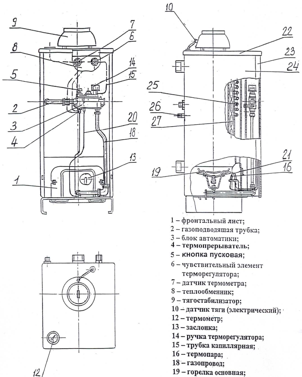
Рис.1. Конструкция аппарата (на виде спереди съёмная панель условно не показана)
