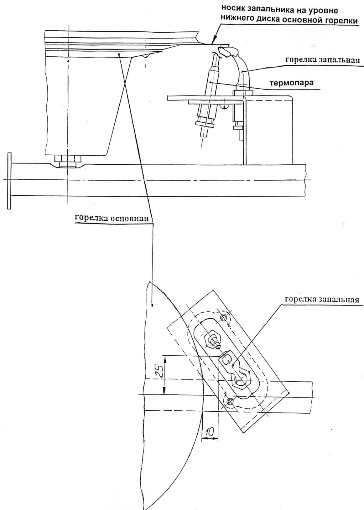
Рис. 7. Схема расположения горелки запальной относительно основной
