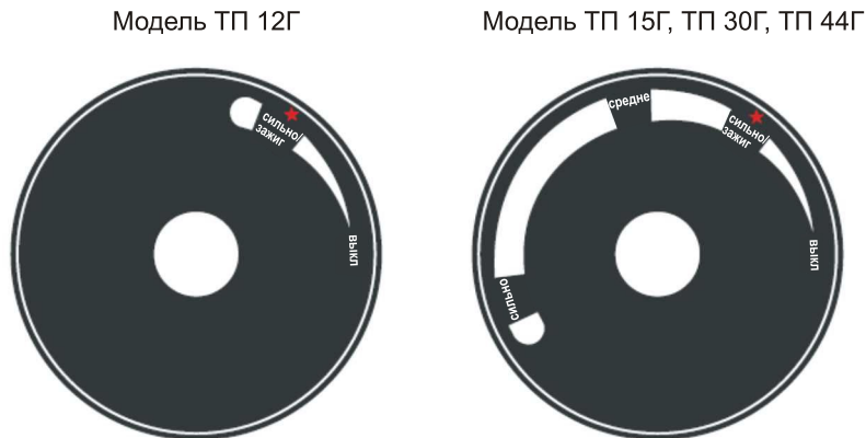
Рис 3. Обозначение положений газового вентиля тепловой пушки
